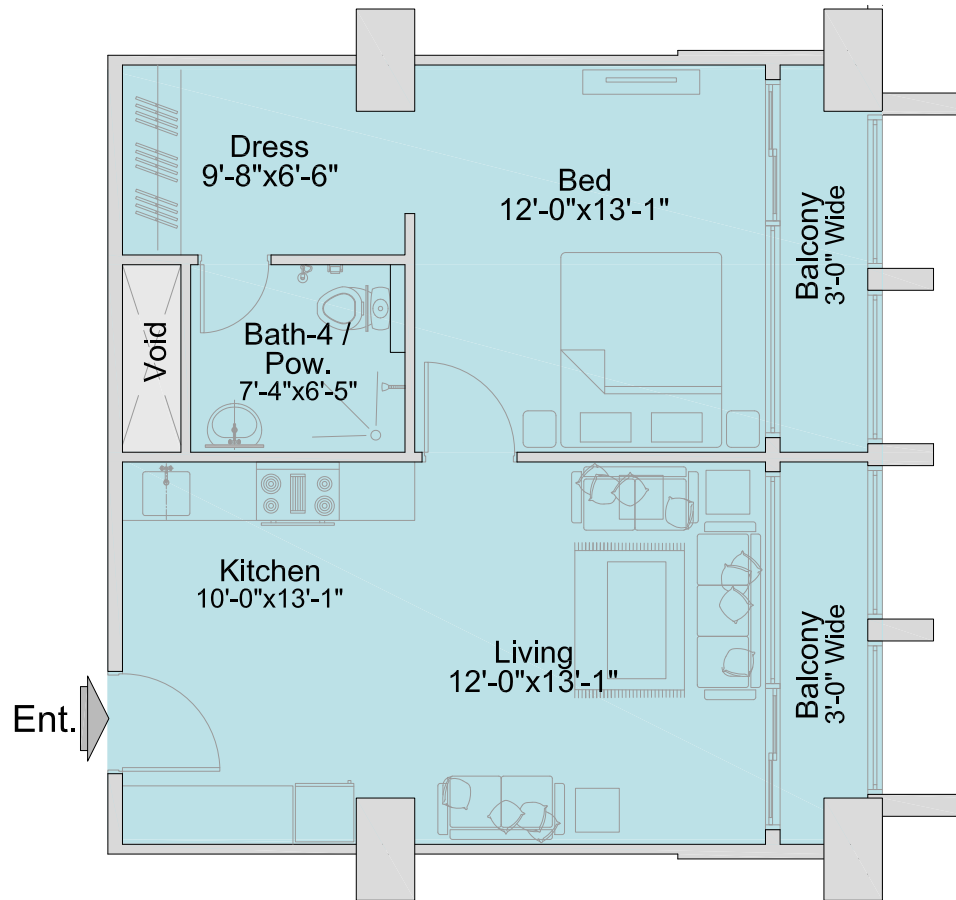
TYPE D1 - 1 BED
